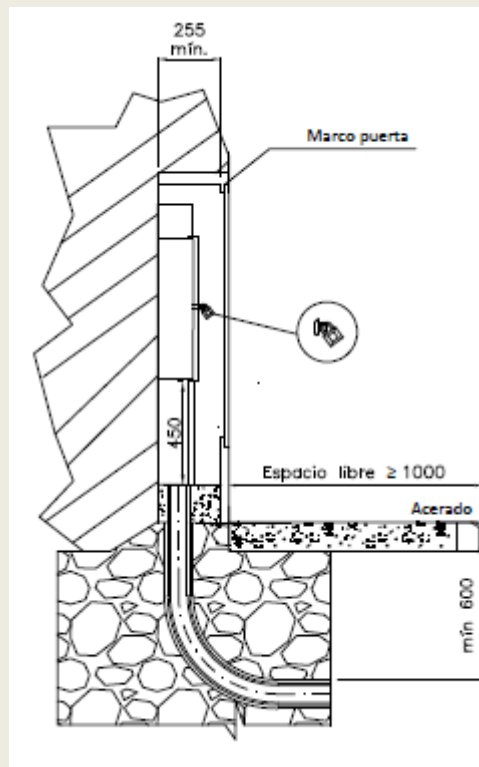
Instalación CGP y CS montaje horizontal. Perfil.
