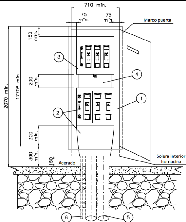
Instalación CGP y CS montaje vertical. Alzado.
