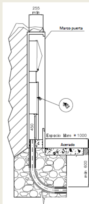
Instalación CPM y CS montaje vertical. Perfil.
