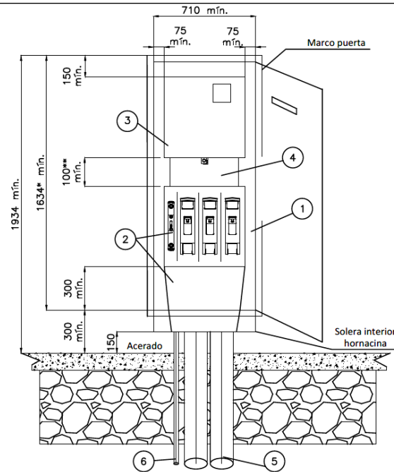
Instalación CPM y CS montaje vertical. Alzado.
