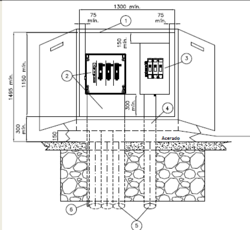
Instalación CGP y CS montaje horizontal. Alzado
