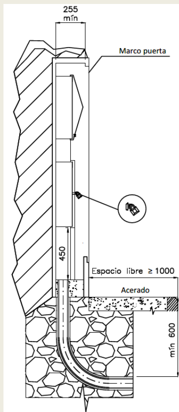
Instalación CGP y CS montaje vertical. Perfil.
